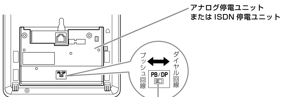
DP(20PPS)/PB 切替スイッチ (アナログ停電用ユニットのみ)
